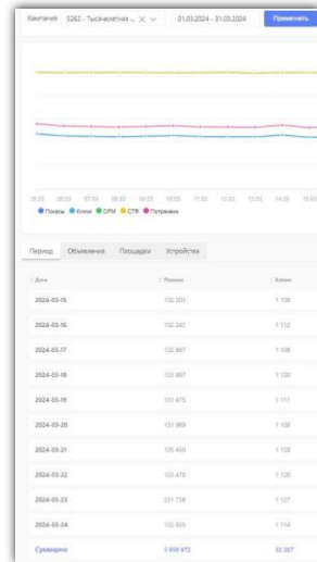
Статистика показов
