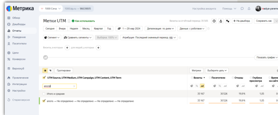
Статистика переходов
